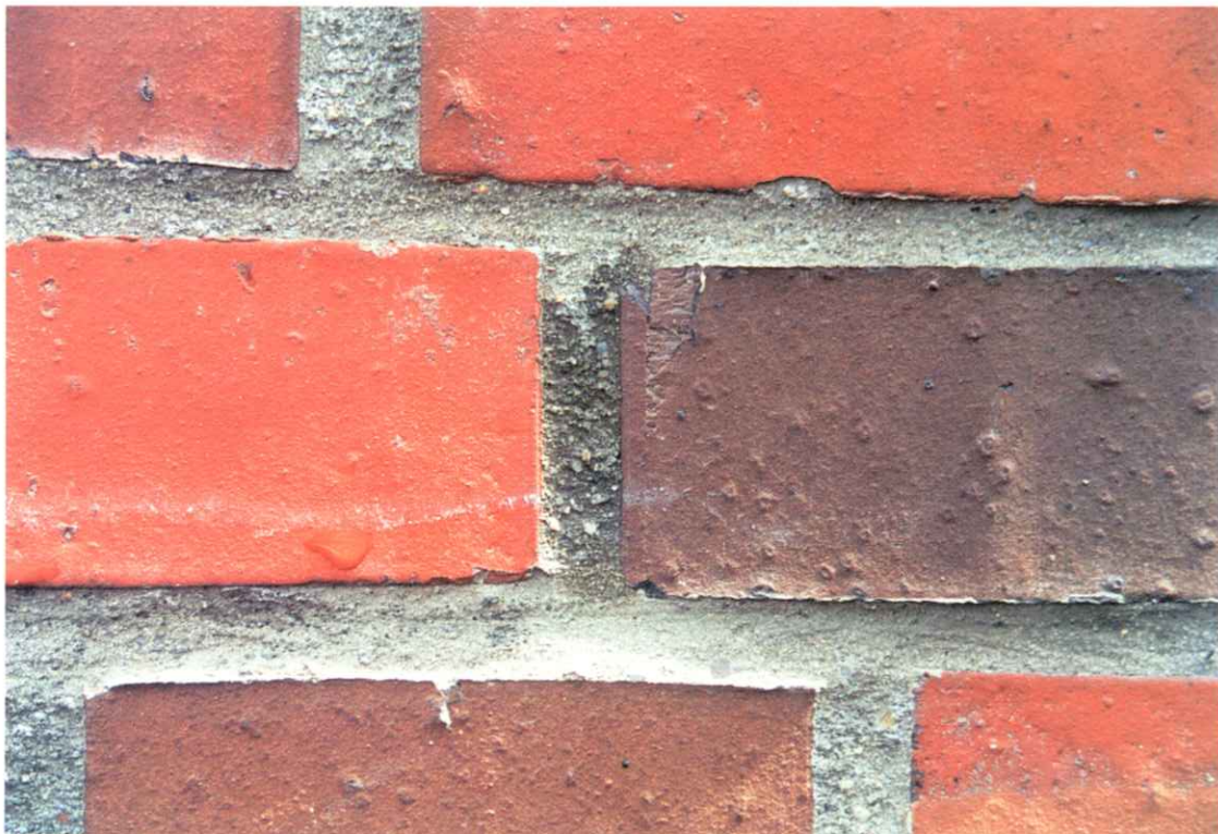
Bild 10: Partiiell fehlende hydrohobe Wirkung des Mörtels
